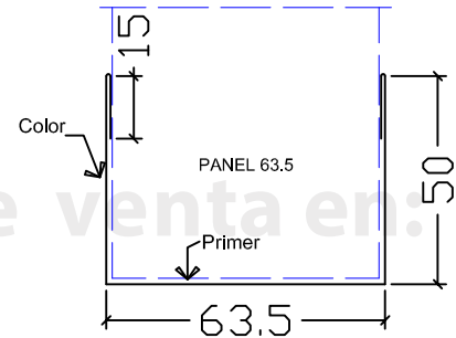
M-3. CANAL U SUPERWALL 2 ½" CALIBRE 20 D = 194 mm.
