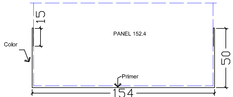
M-7. CANAL U SUPERWALL 6" CALIBRE 20 D = 284mm.
