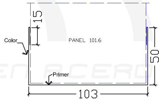
M-5. CANAL U SUPERWALL 4" CALIBRE 20 D = 233 mm.
